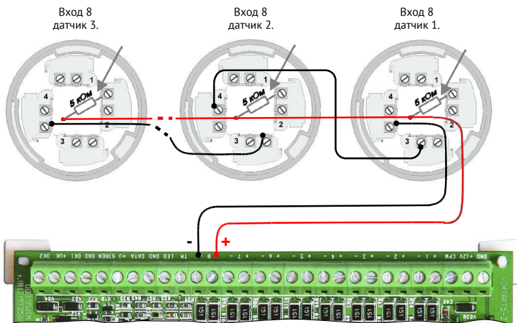
Рисунок 44. Схема подключения пожарных датчиков на вход №8
