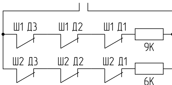
Рисунок 43. Эквивалентная схема для рис. 45
