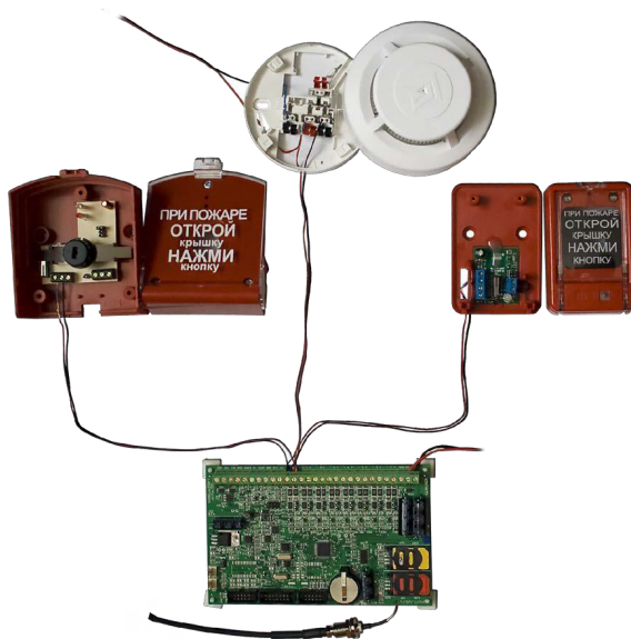
Рисунок 49. Фотография подключения пожарных датчиков
