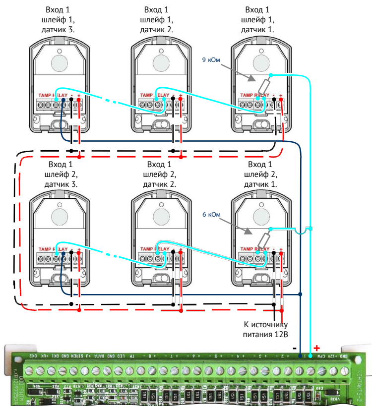
Рисунок 42. Схема подключения охранных датчиков на вход №1
