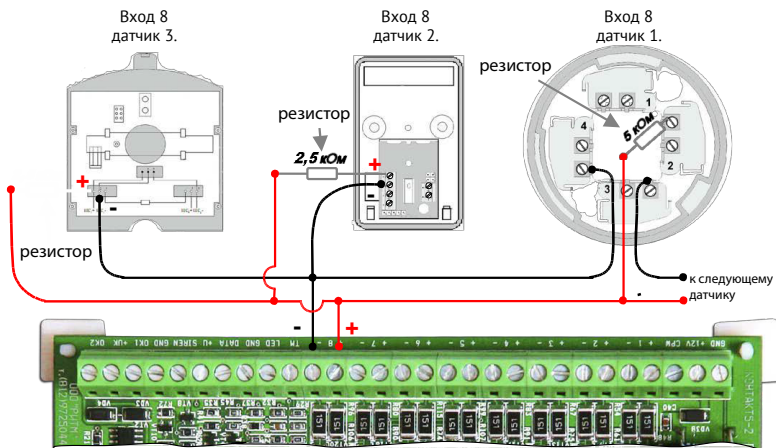
Рисунок 47. Схема подключения пожарных датчиков на вход №8
