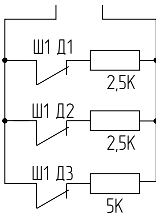
Рисунок 48. Эквивалентная схема для рис. 50
