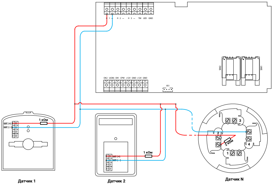
Рисунок 11. Схема подключения ручных пожарных извещателей
