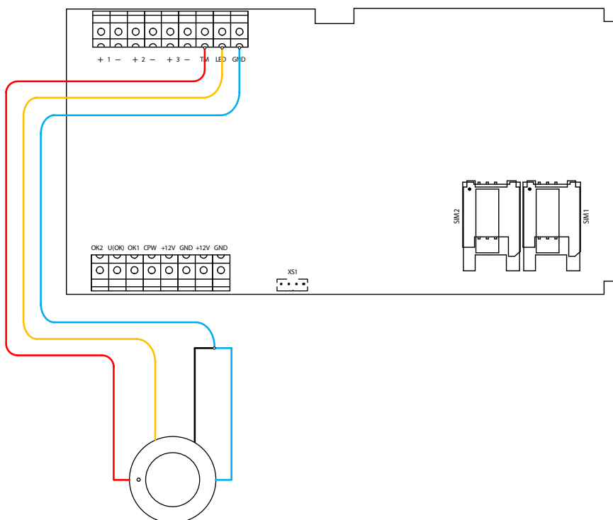
Рисунок 12. Схема подключения считывателя ТМ
