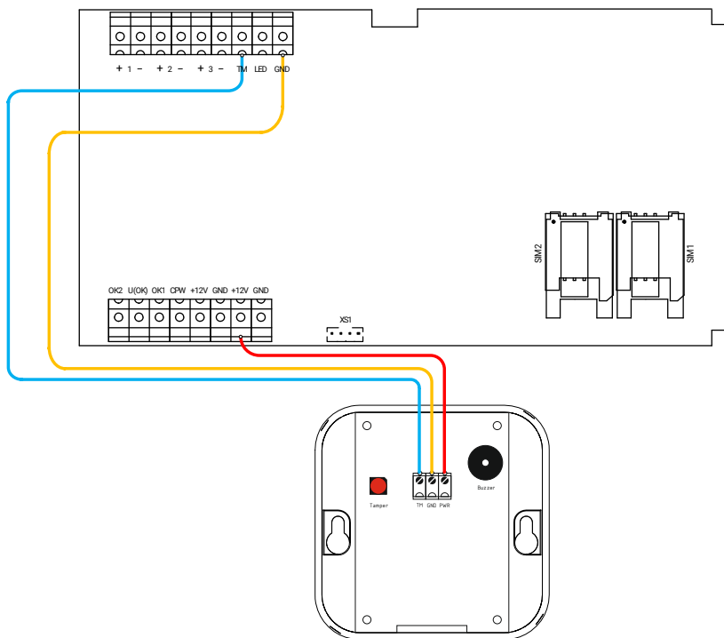
Рисунок 17. Схема подключения клавиатуры KB2-3
