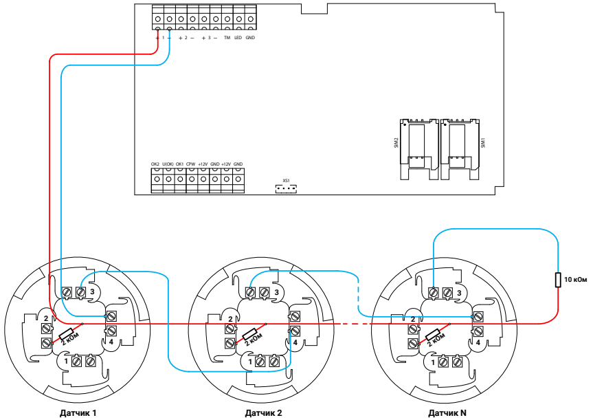
Рисунок 10. Схема подключения пожарных шлейфов с контролем обрыва
