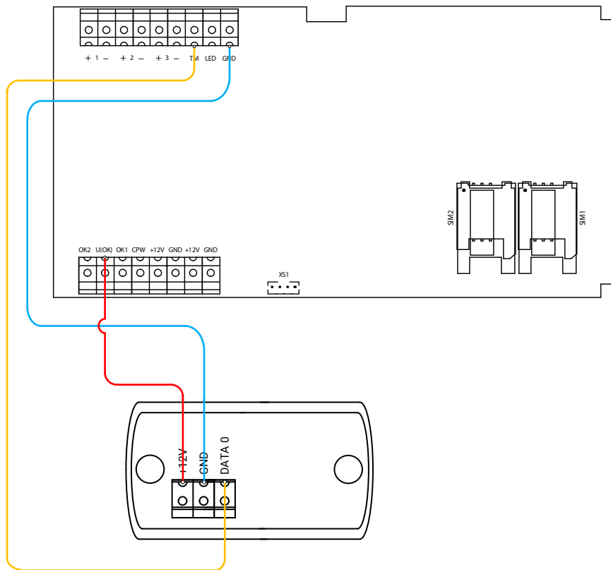
Рисунок 14. Схема подключения считывателя «Matrix-II»
