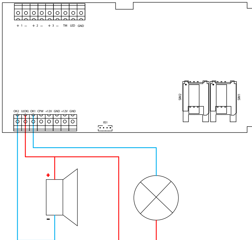
Рисунок 16. Схема подключения исполнительных устройств
